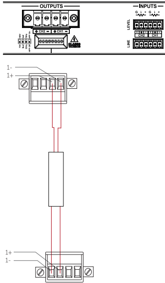
Figure 4.2: Bias D1
